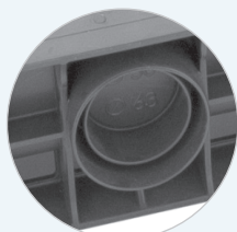
Scarichi laterali H 7,5: scarico Ø 50 - 63 H15: Scarico Ø 80 - 100 - 110
